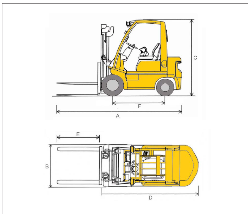
Abmessungen
