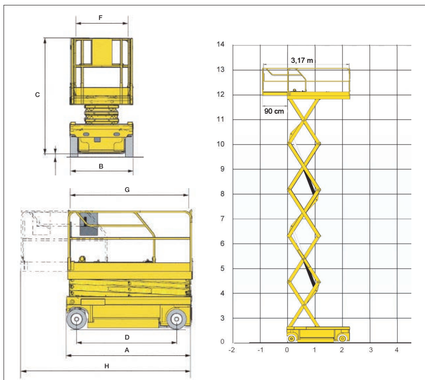
Abmessungen
