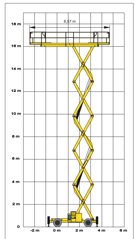
Abmessungen
