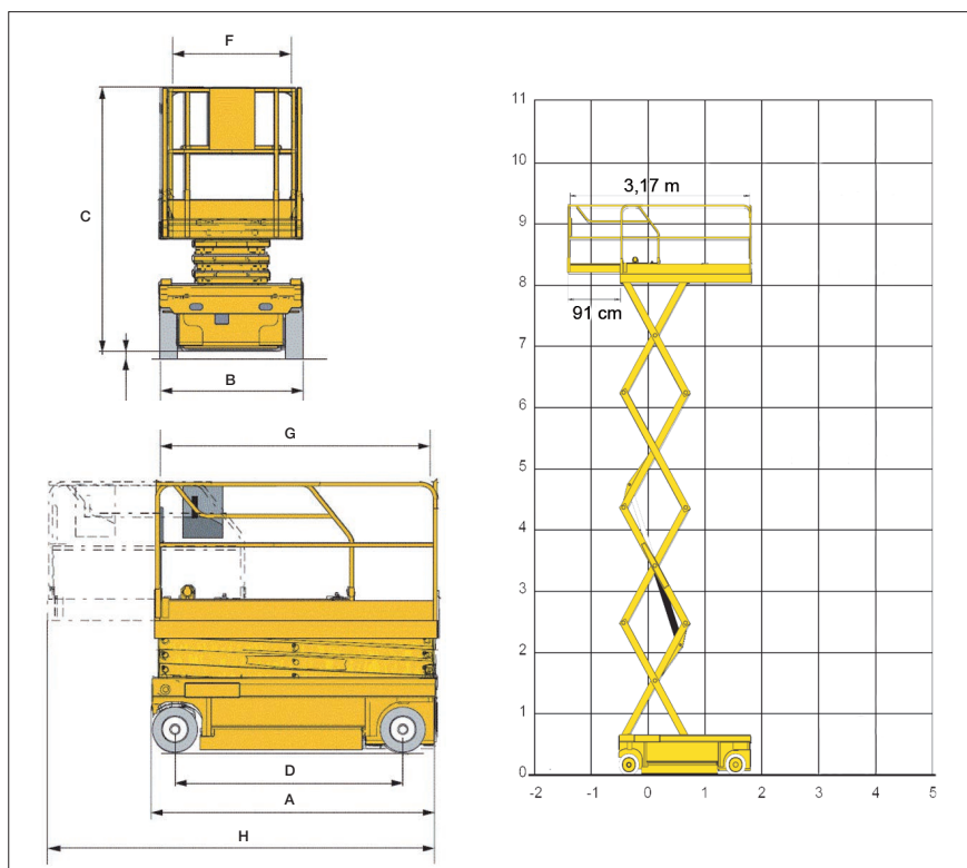
Abmessungen
